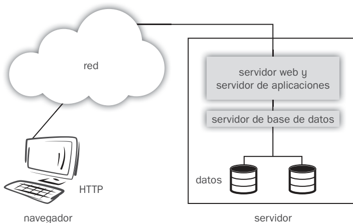
Figura 9.7. Arquitectura de aplicación web en dos capas.
