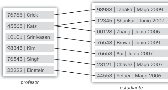
Figura 7.20. fecha como un atributo del conjunto de entidades estudiante .
