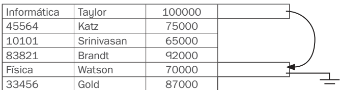
Figura 10.15. Estructura de archivo en agrupaciones de varias tablas con cadenas de punteros.
