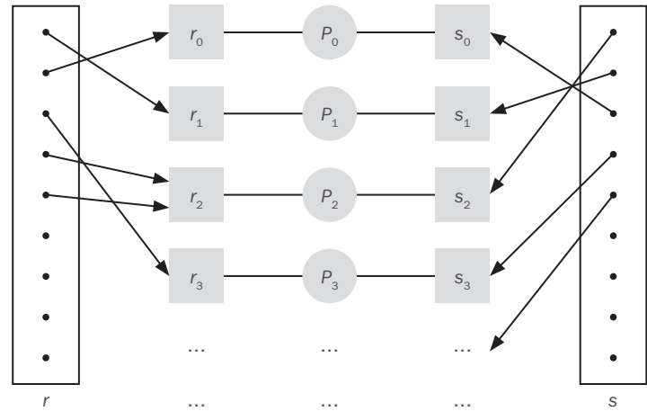
Figura 18.2. Reunión por división paralela.
