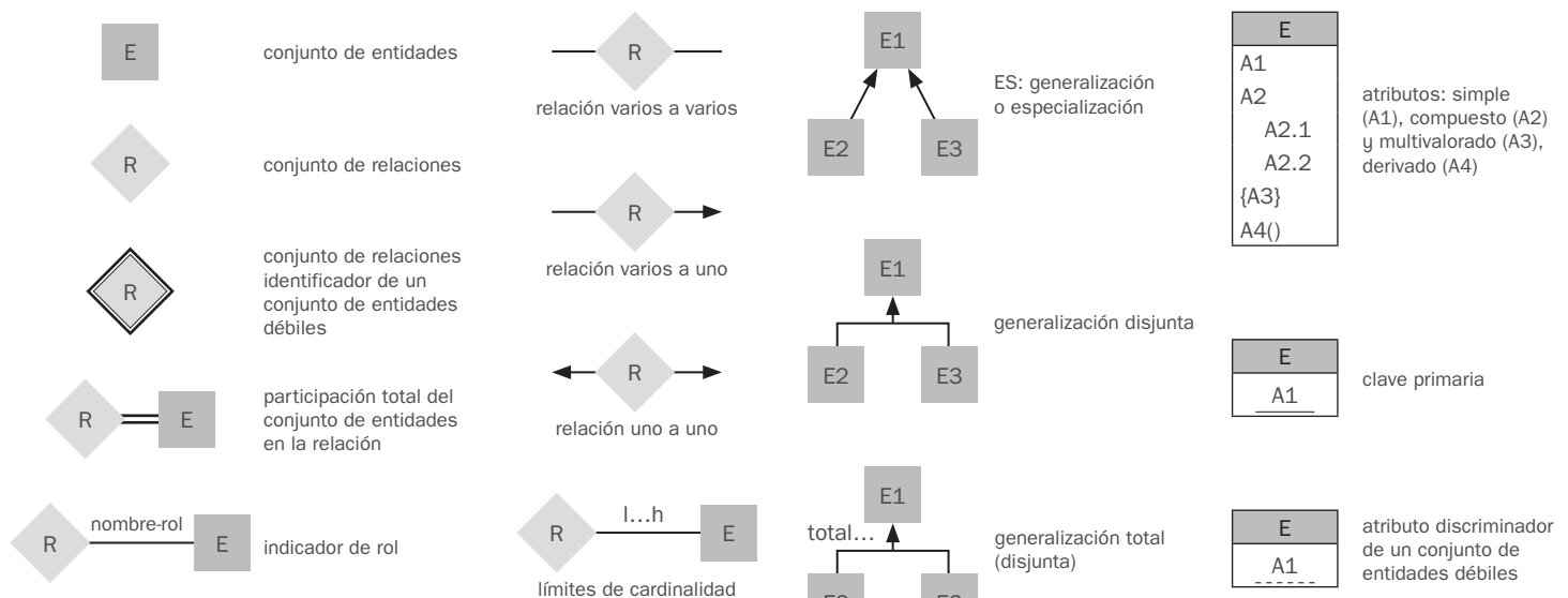
Figura 7.24. Símbolos usados en la notación E-R.
