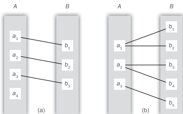
Figura 7.5. Correspondencia de cardinalidades (a) Uno a uno. (b) Uno a varios.
