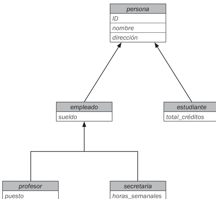
Figura 22.7. Especialización y generalización.
