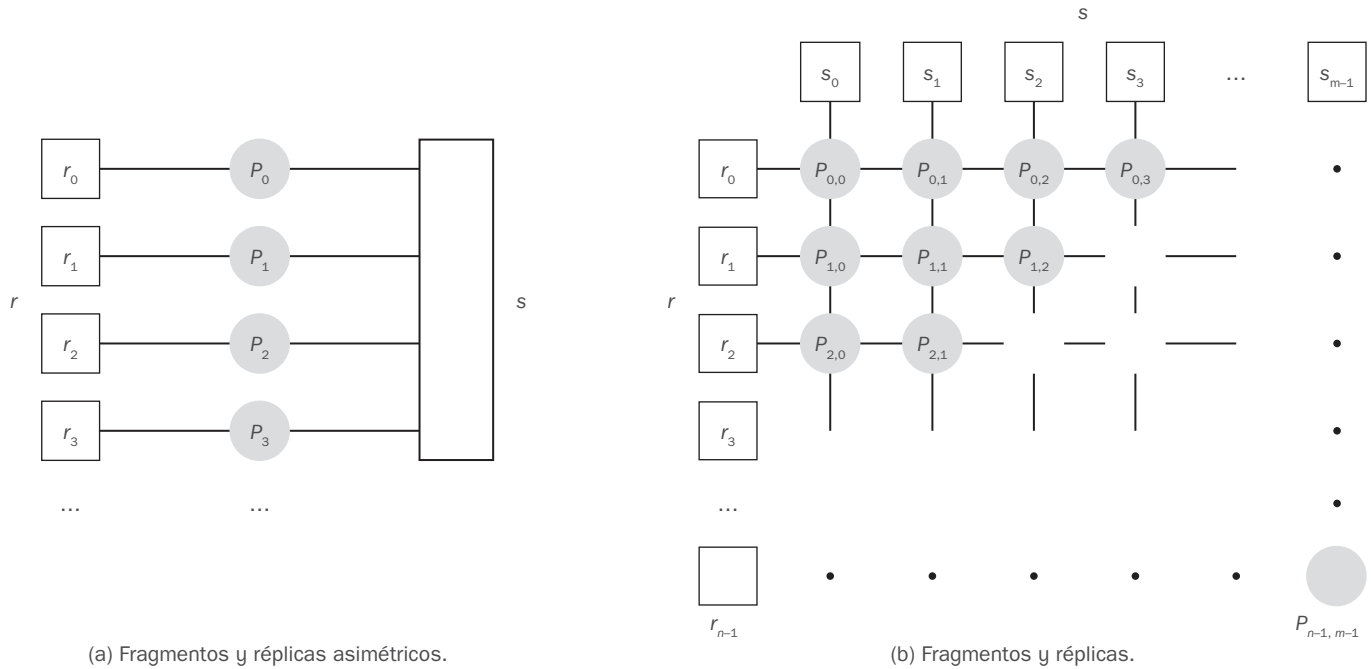
Figura 18.3. Esquemas de fragmentos y réplicas.
