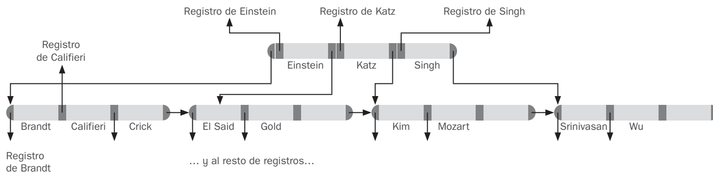
Figura 11.21. Árbol B equivalente al árbol B^+ de la Figura 11.13.
