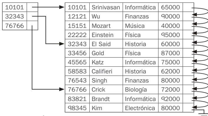
Figura 11.3. Índice disperso.
